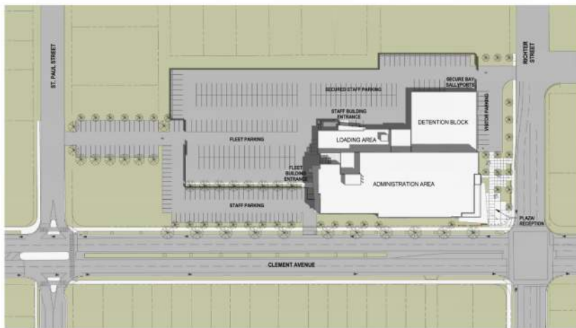
4 SITE PLAN SCALE: 1:750
